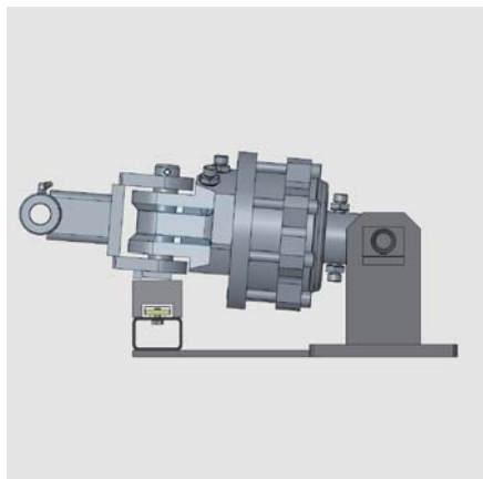
Drehkopf-Umlegevorrichtung
